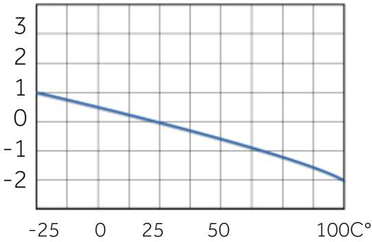
Delta C/C %
