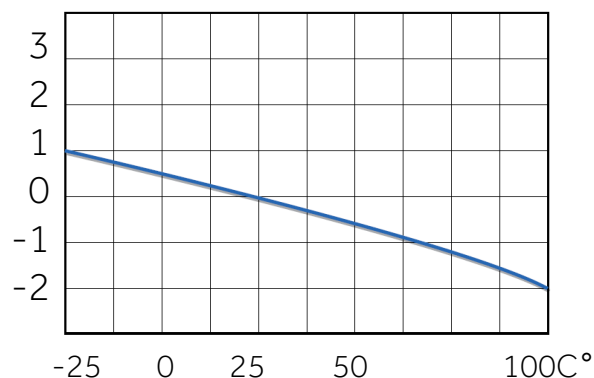
Delta C/C %
